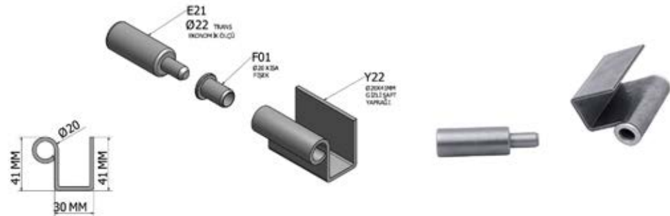
Y22 Ø20x41 MM ŞAFT KAPI MENTEŞESİ GİZLİ YAPRAK
